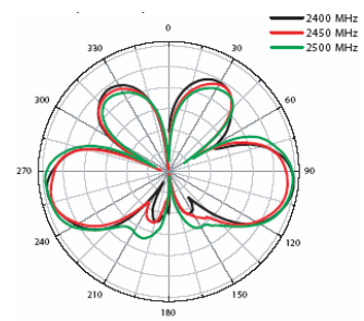
Vertical (V Plane)
